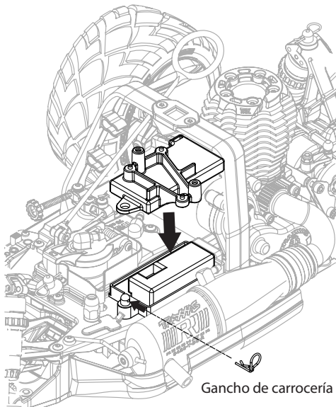
Gancho de carrocería
